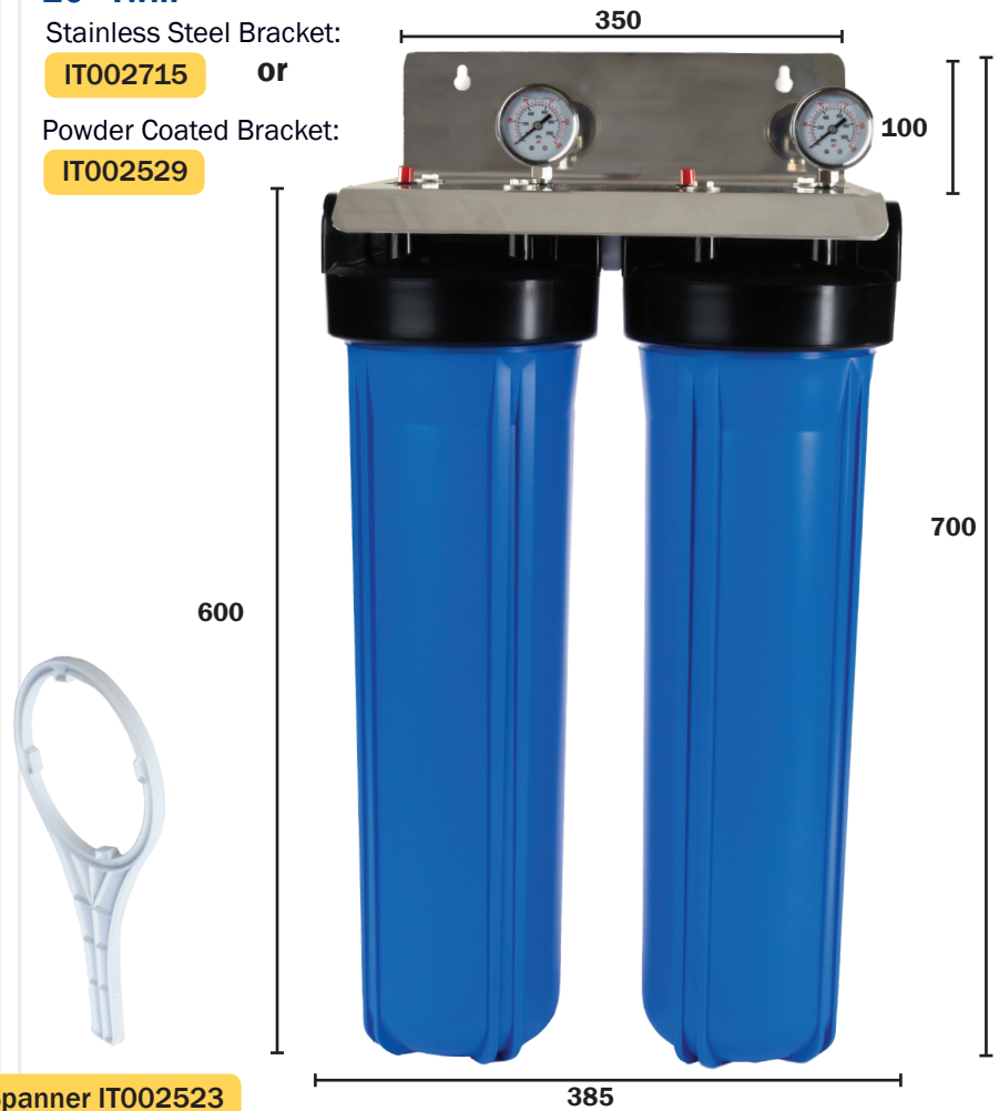
385mm W x 700mm H x 205mm D
